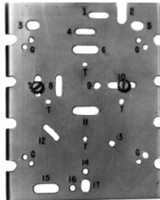
Subplate (See note.)
