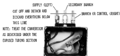
Subplate (See note.)
