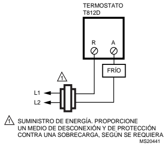
Fig. 8. T812D en aplicación de enfriamiento únicamente.
