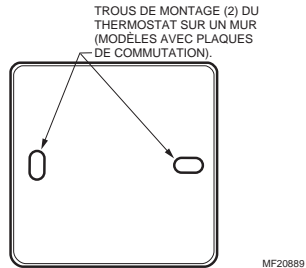
Fig. 3. Emplacement des trous de montage sur les modèles avec plaque de commutation.
